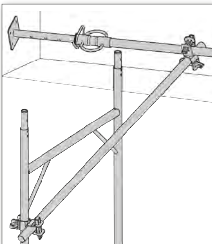
Ancrage par étançons :
