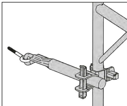
Ancrage par chevillage
