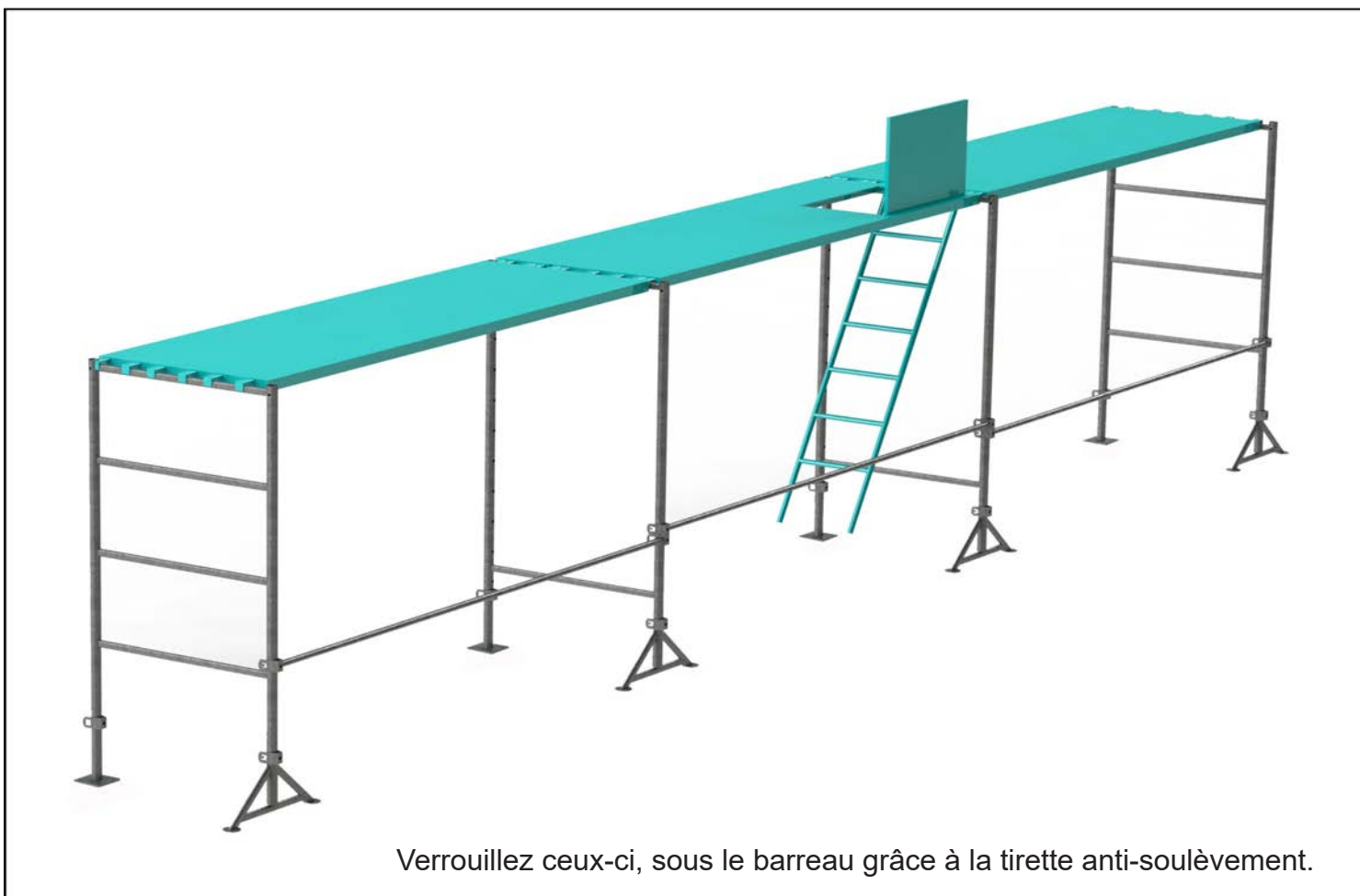
Configuration 2 : À 2 m du sol, installez l'échelle d'accès, sous le plancher trappe
