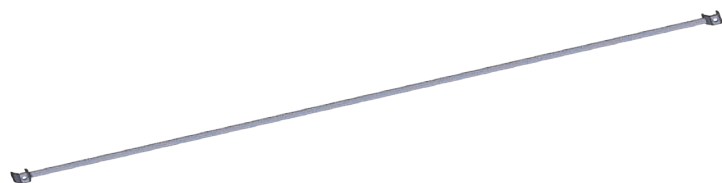
LISSE ENTRETOISE Longueur : 3 m Réf : ES49014
